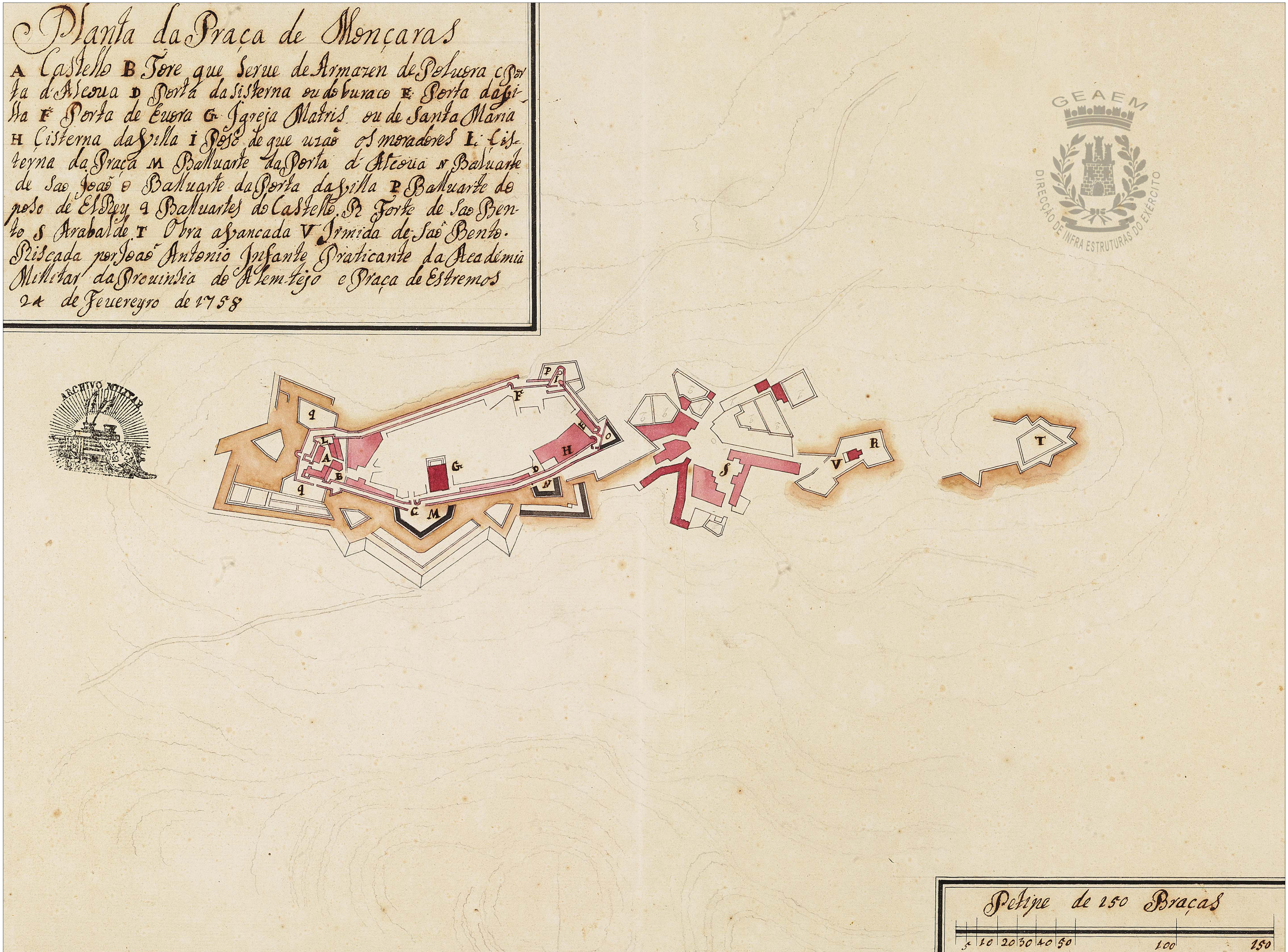
joão antónio - planta da praça de monçaras - 1758. fonte: direcção de infraestruturas do exército
