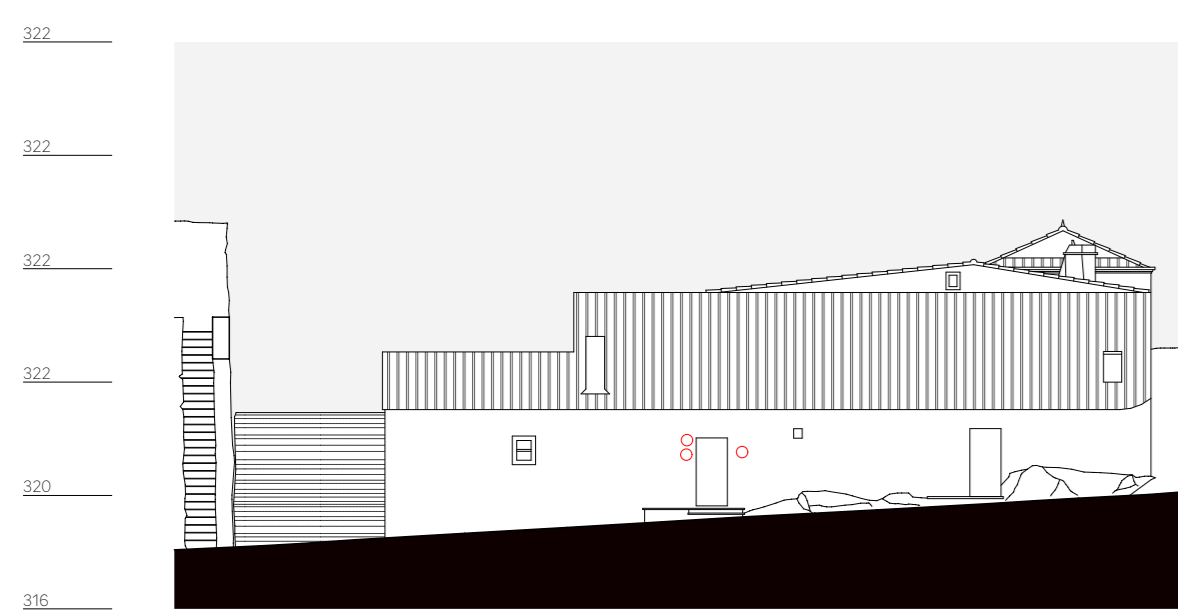
quarteirão T, alçado 1, rua dos celeiros n. 10
