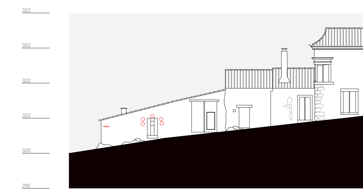
quarteirão T, alçado 4, rua dos celeiros n. 2 a 8
